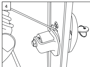
Intensives Ölen des Schließsystems durch die zwei innenliegenden eckigen Öffnungen oberhalb und unterhalb des Schließzylinders. / Intensive oiling of the locking system through the two internal angular openings above and below the locking cylinder.
